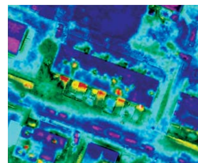
SUR CETTE THERMICARTE® LES TOITS ROUGES SONT ENVIRON 10° PLUS CHAUD QUE L'AIR AMBIANT, PREUVE D'UNE DÉPERDITION IMPORTANTE DE CHALEUR
